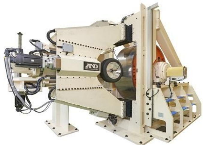
動的接地力試験機 DCFR
