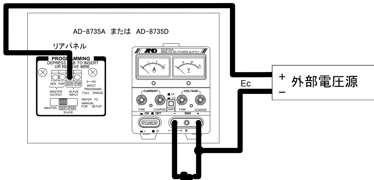
図5-3 外部電圧による出力電圧のコントロール
