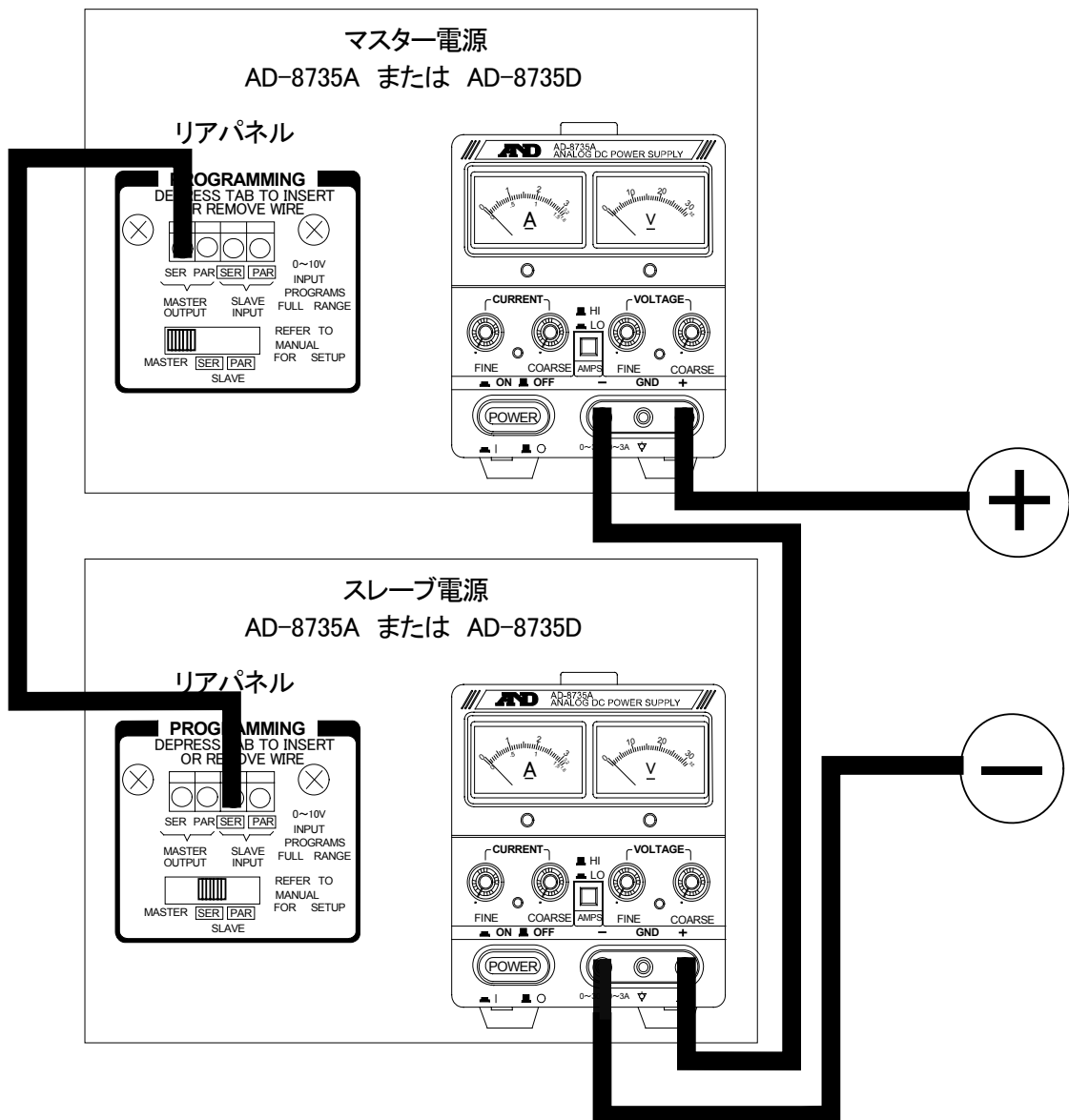
図5-1 直列接続
