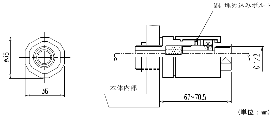
図2 引込器具
