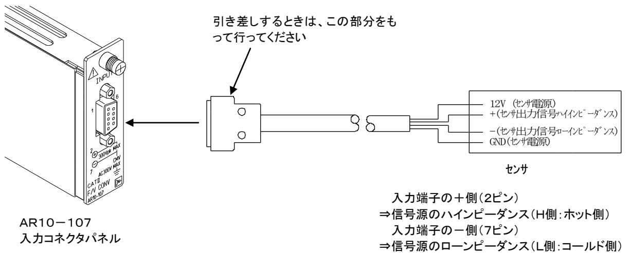
図3-1: 入力ケーブルの接続
