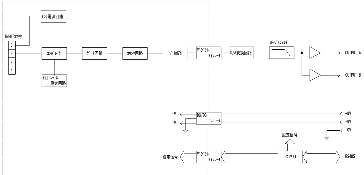
図5-1 ブロック図
