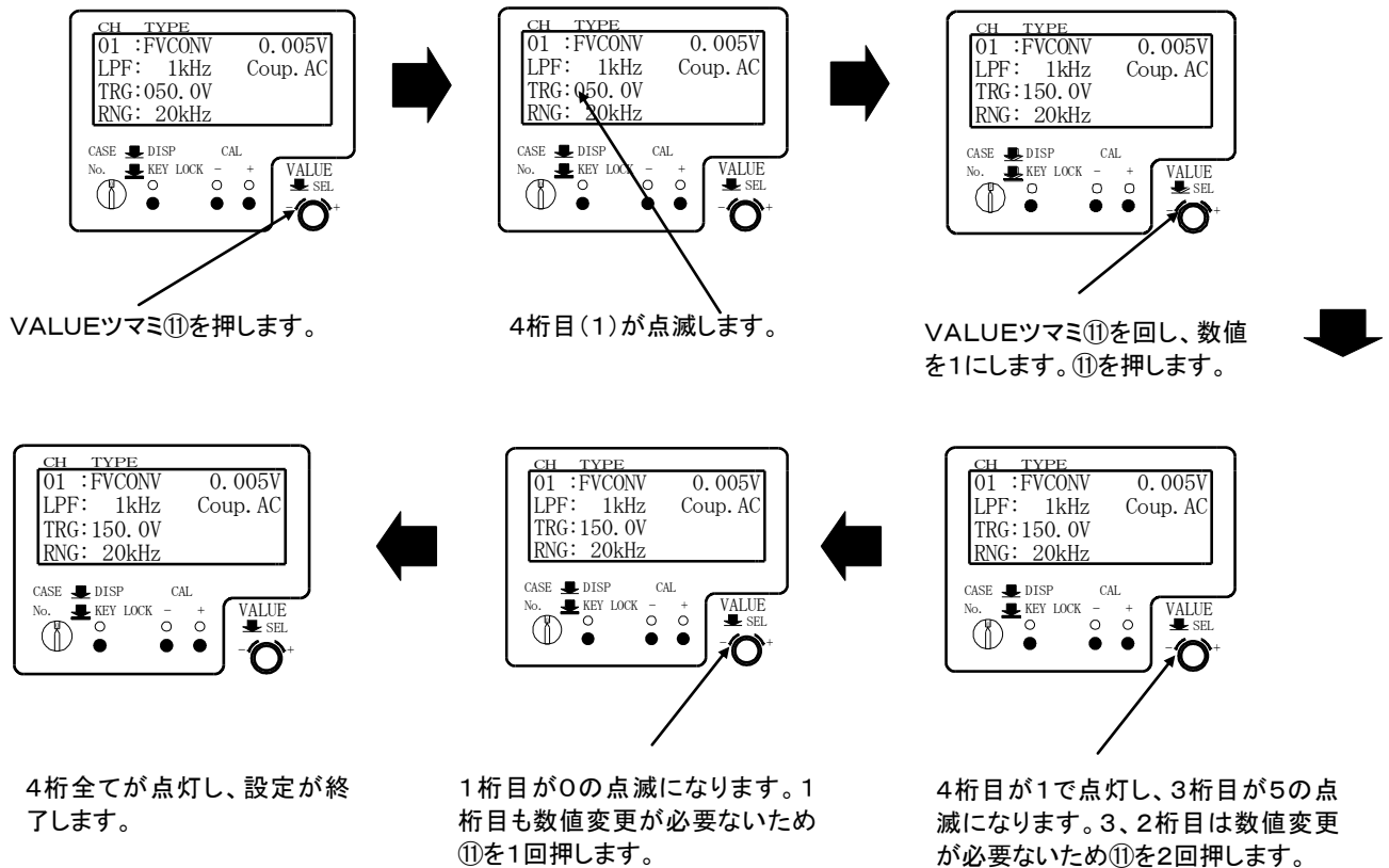
図2-2:トリガレベル設定値
