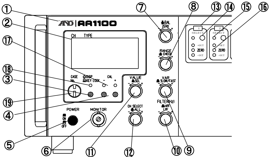
図2-1: 本体前面
