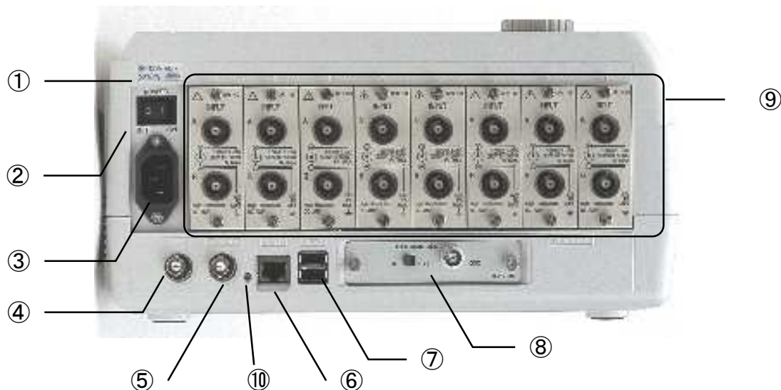
(上図は2CH高速DCアンプユニット 8スロット 構成の時の入カスロット部)
