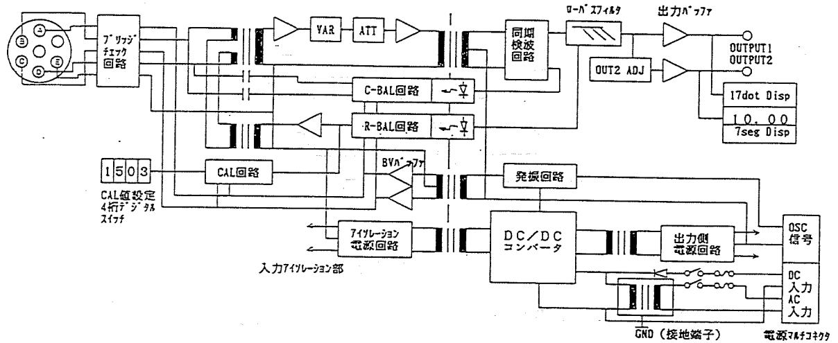
図 23 ブロック図
