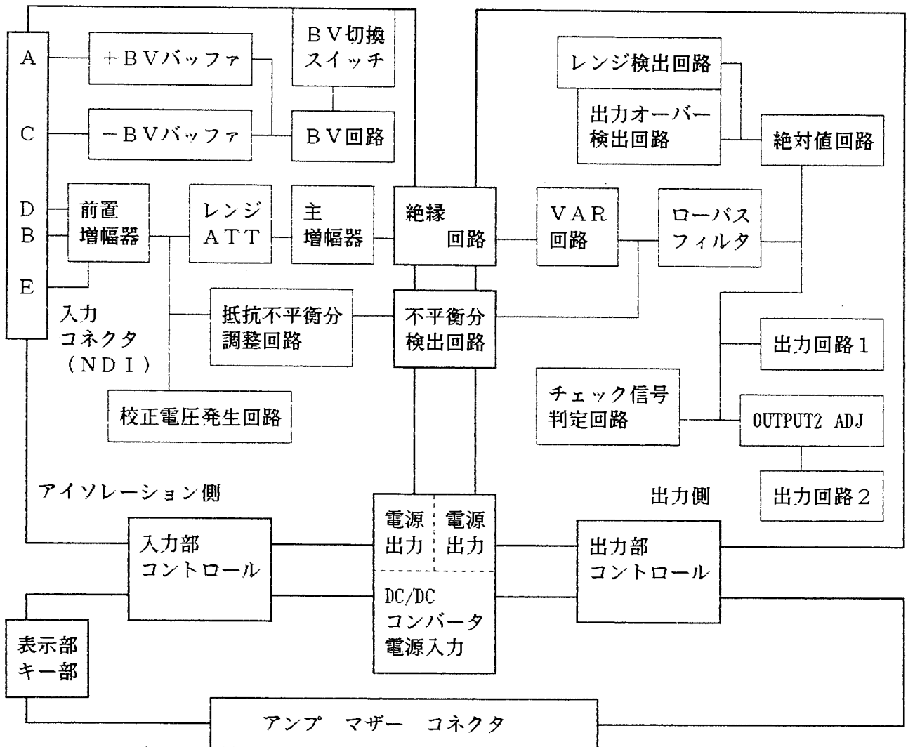
ブロック図
